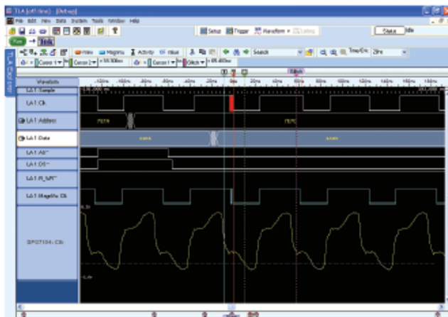
图 14. MagniVu™ 采集显示时钟信号上的毛刺。
