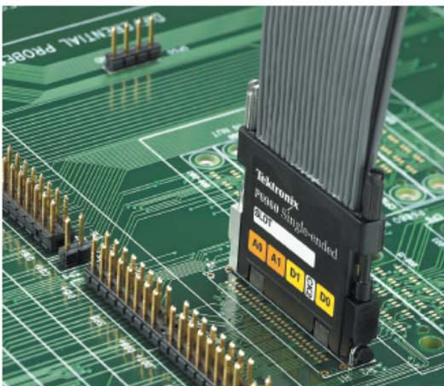
图 6. D-Max™ 无连接器分析仪探头。
