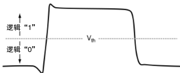
图 2. A 逻辑分析仪确定相对于门限电压电平的逻辑值。
