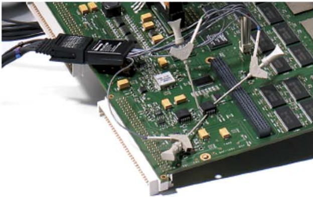
图 4. 通用探头。
