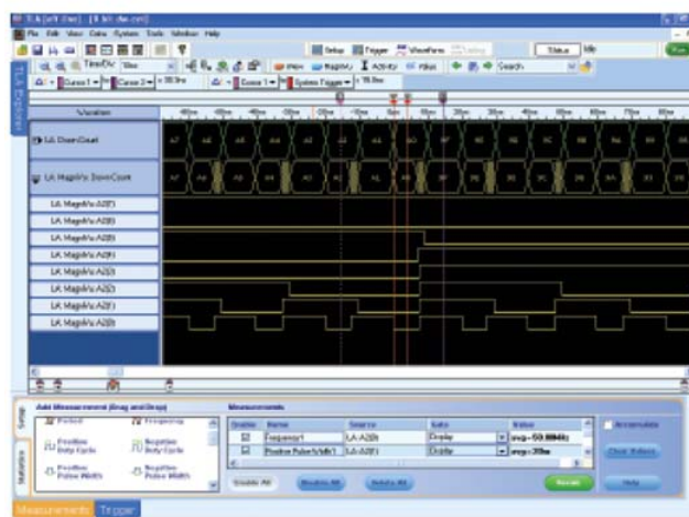
图 21. 自动测量改善了工作效率。
