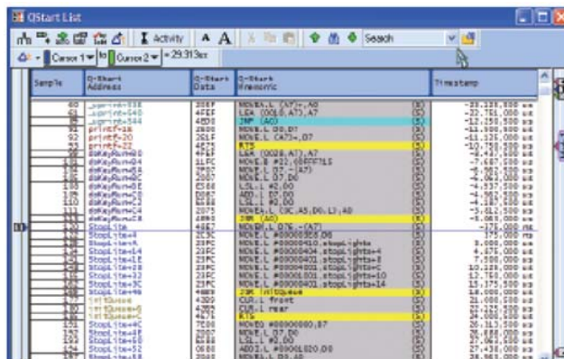
图 19. 实时命令追踪显示画面。
